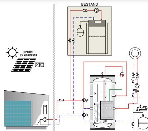
Nachrüstlösung AEROTOP® SG mit Pufferspeicher und FRIWA
